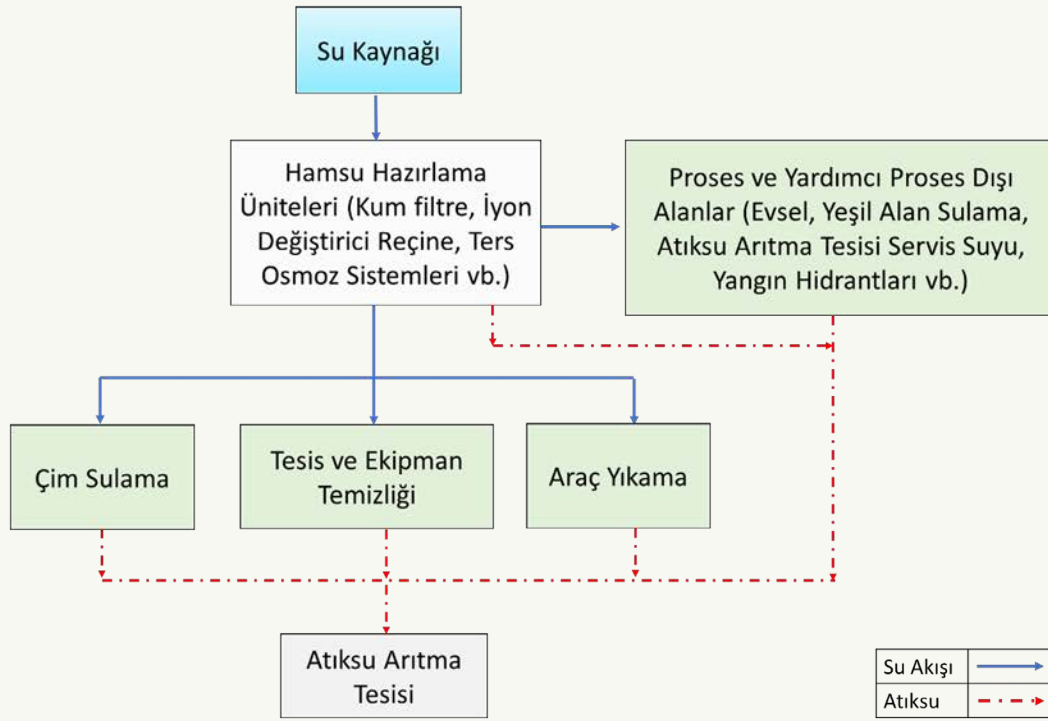
Spor Kulüplerinin Faaliyetleri Sektörü Su Akım Şeması
