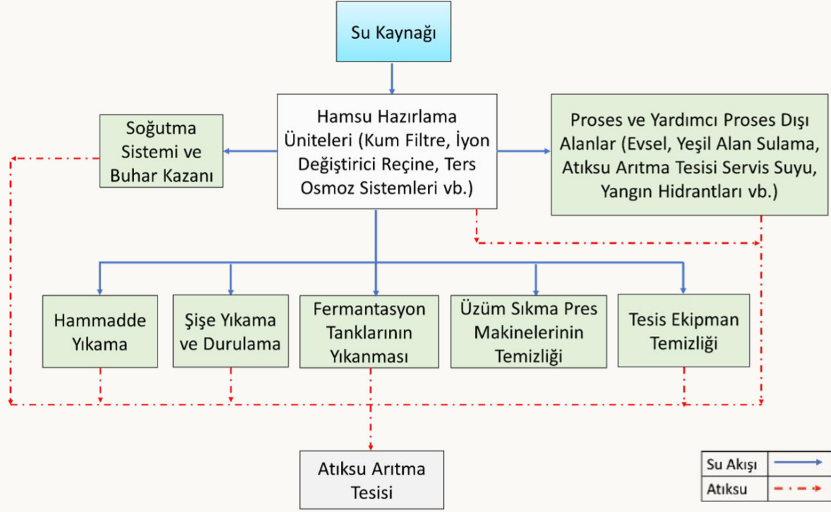
Üzümden Şarap İmalatı Su Akım Şeması
