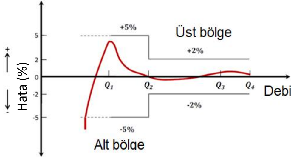
Yeni bir su sayacının hata eğrisi
