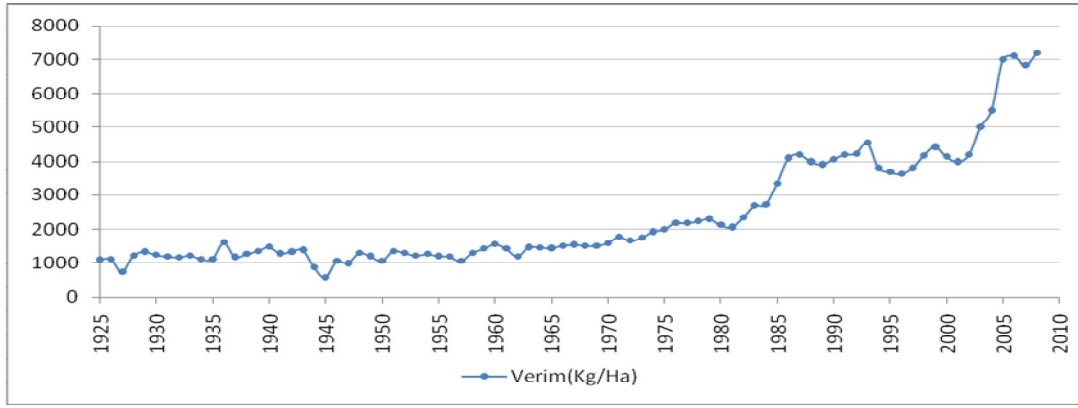
Şekil 3: Mısır Verimi
