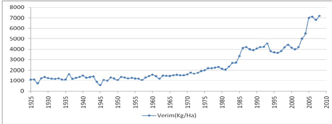
Şekil 3: Mısır Verimi
