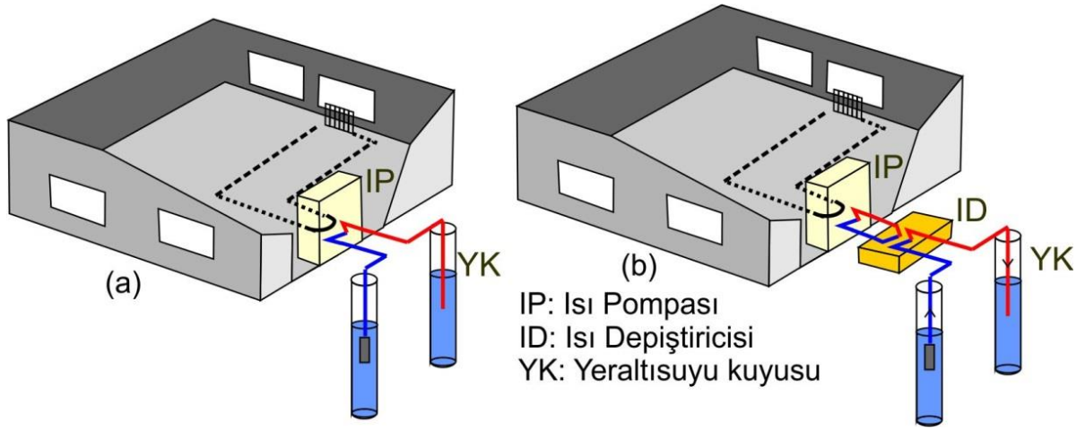
Şekil 5 - Yeraltısuyu kaynaklı ısı pompası sistemi: Yeraltısuyunun (a) ısı pompasından ayrı olmayan, (b) ısı pompasından ayrı olan
