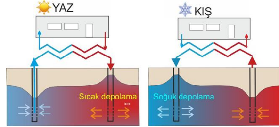
Şekil 2 - Akiferde Termal Enerji Depolama (ATED) Sistemi
