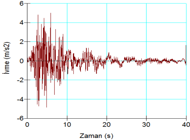
řekil 3 - Loma Prieta depremi ölçeklenmiř ivme kaydı.
